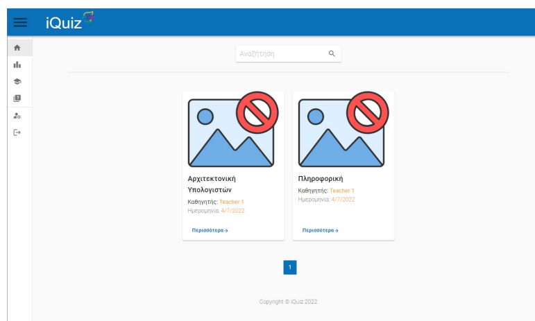
Εικόνα 79: Αρχική σελίδα
