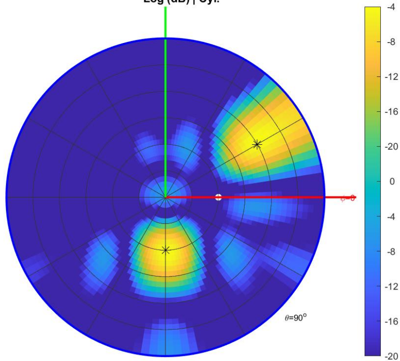
Εικόνα 26 : Διάγραμμα Beam Splitting 2 δέσεων
