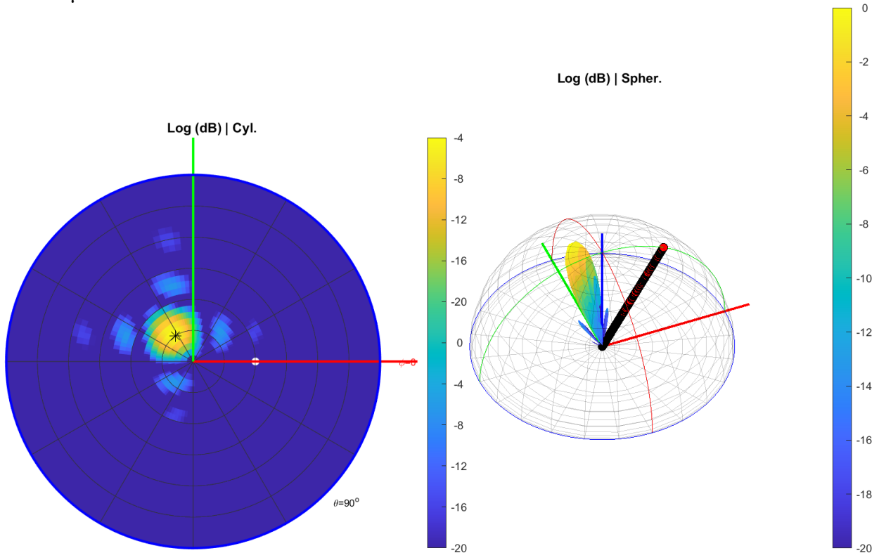
Εικόνα 20: Διάγραμμα ακτινοβολίας Beam Steering
