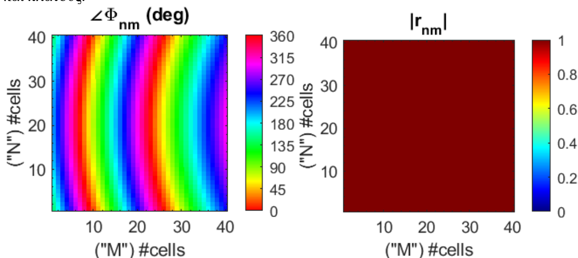
Εικόνα 30: Φάση και πλάτος μεταεπιφάνειας για σφαιρικό κύμα (NF2FF)
