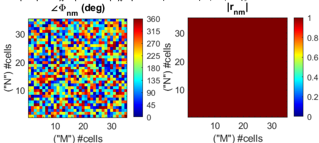
Εικόνα 66: Φάση και πλάτος σφαιρικού κύματος για diffused scattering
