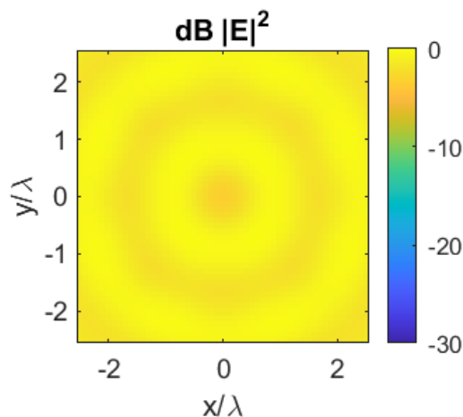
Εικόνα 48: Διάγραμμα ακτινοβολίας για εστίαση σφαιρικού κύματος πολύ κοντά στην μεταεπιφάνεια
