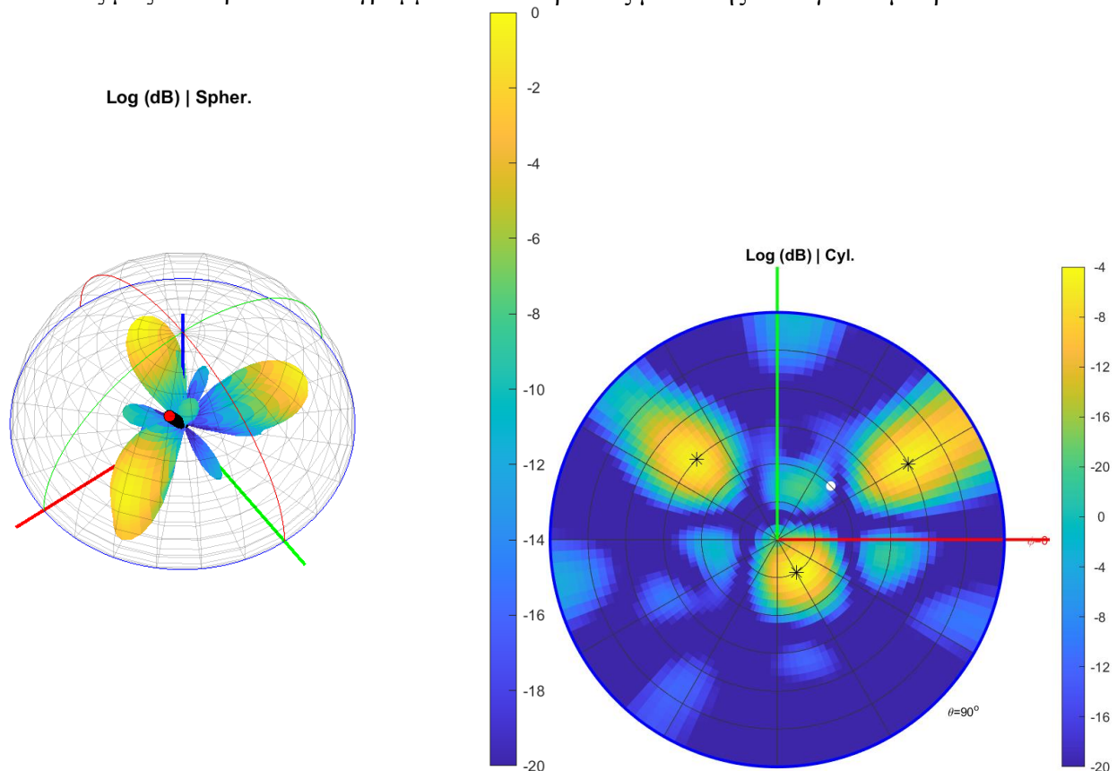
Εικόνα 61: Διάγραμμα ακτινοβολίας beam splitting 3 λοβών για επίπεδο κύμα
