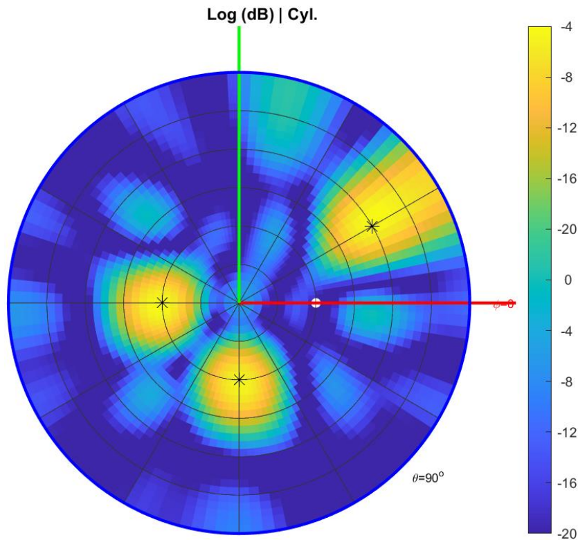
Εικόνα 28: Διάγραμμα ακτινοβολίας Beam Splitting 3 λοβών
