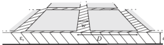
Εικόνα 14: Η απορροφητική δομή. Δεν υπάρχουν ενσωματωμένα μεταλλικά πτερύγια στο υπόστρωμα.
