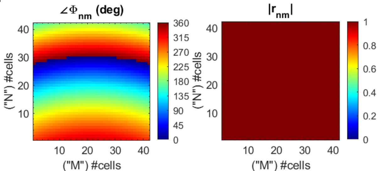
Εικόνα 54: Προφίλ φάσης και πλάτους μεταεπιφάνειας για ανακατεύθυνση δέσμης σφαιρικού κύματος
