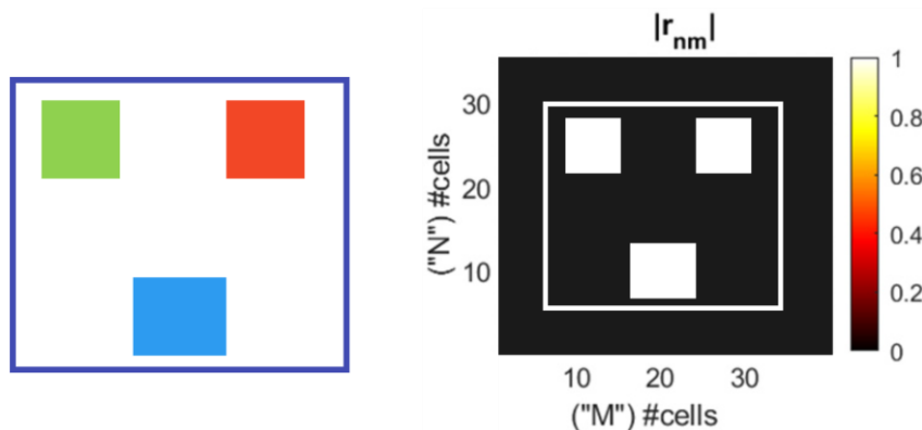
Εικόνα 71: Point Cloud που θέλουμε να αναπαράγουμε στο Image/Focal Plane και μετατροπή σε πλάτος.
