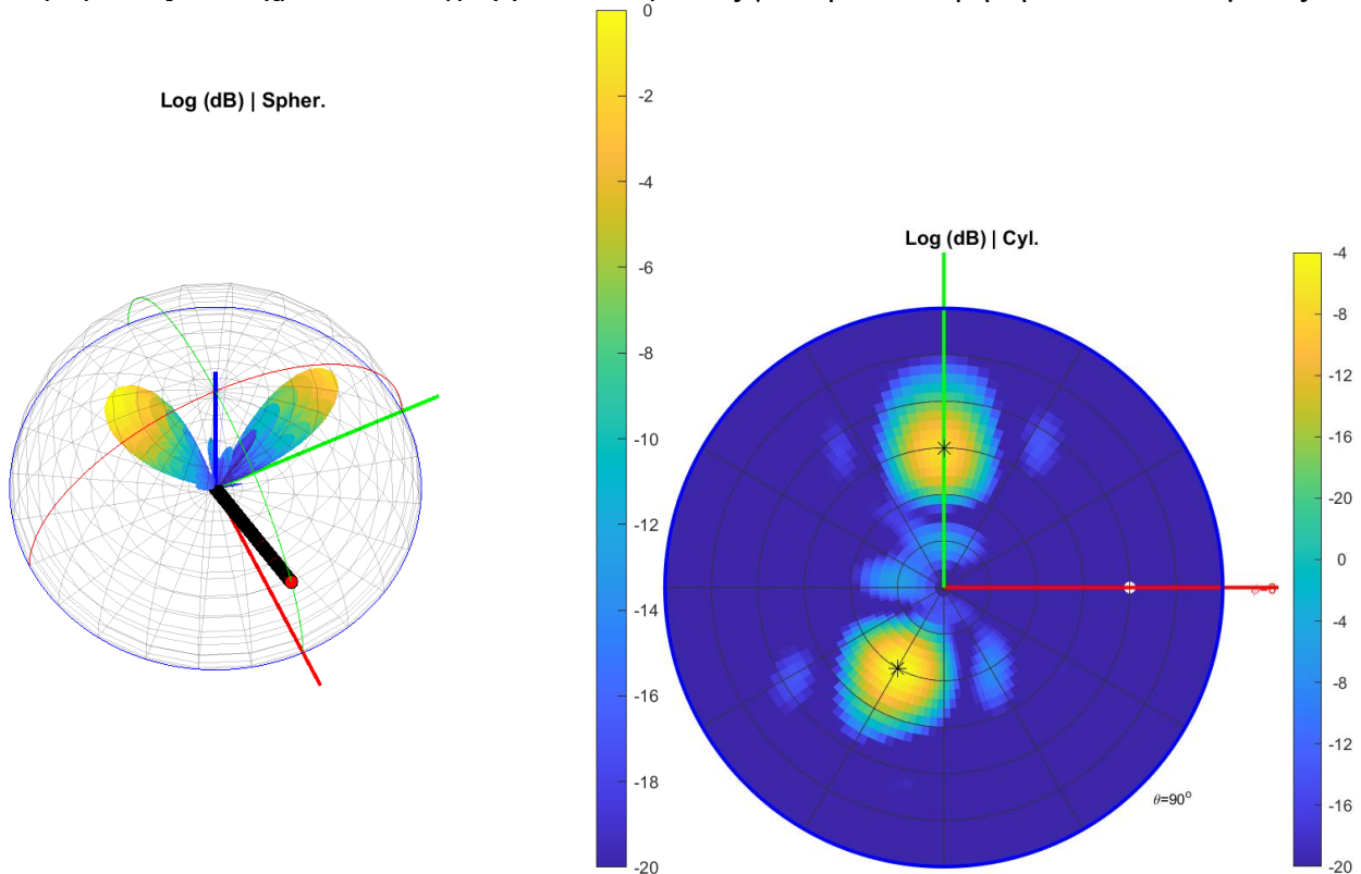
Εικόνα 59: Διάγραμμα ακτινοβολίας beam splitting 2 λοβών επίπεδου κύματος σε (\theta, \varphi)=(45,90) και (\theta, \varphi)=(30,240)
