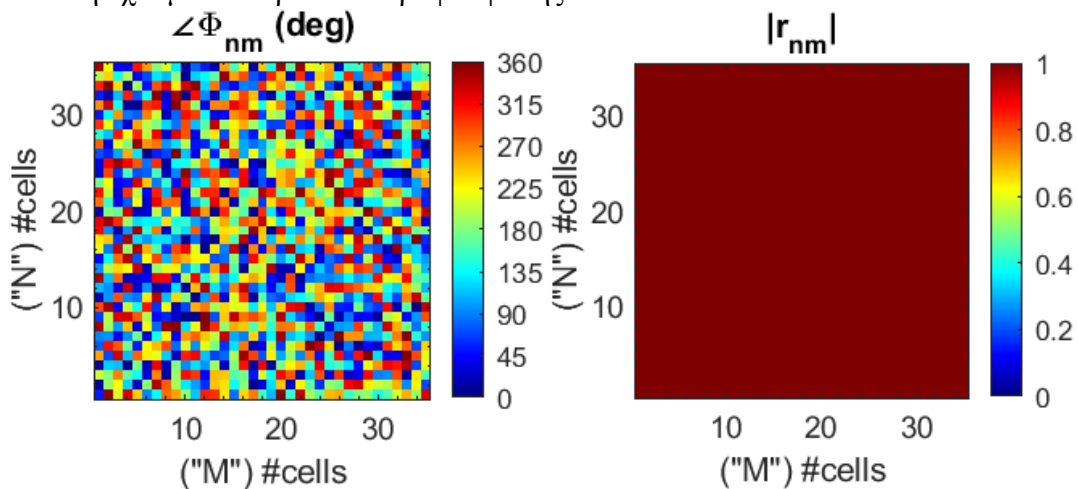
Εικόνα 64: Φάση και πλάτος μεταεπιφάνειας για diffused scattering επίπεδου κύματος.
