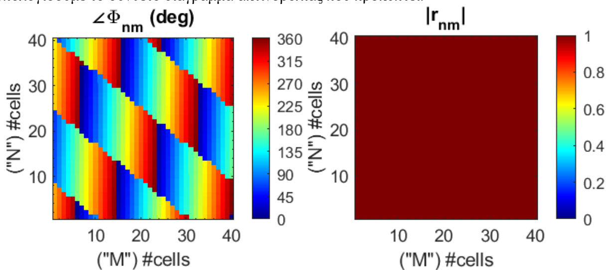
Εικόνα 25: Φάση και Πλάτος Beam Splitting (FF2FF)
