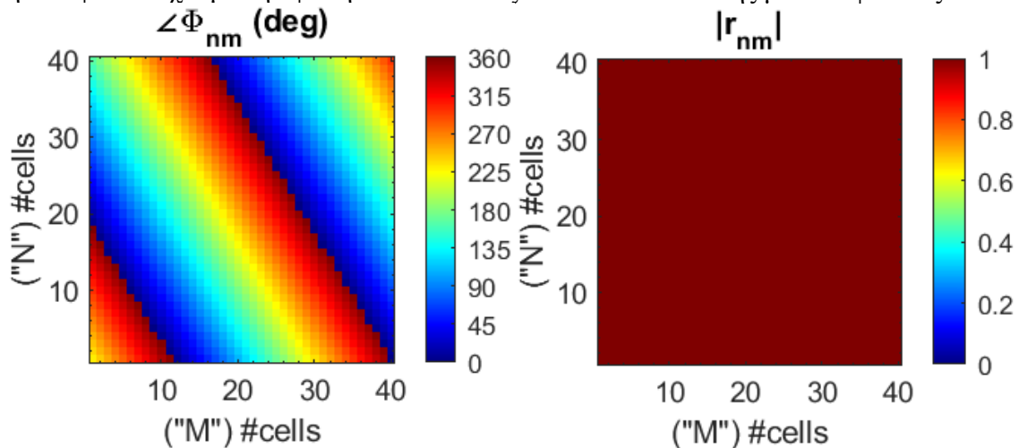
Εικόνα 19 : Φάση και πλάτος M/E beam steering
