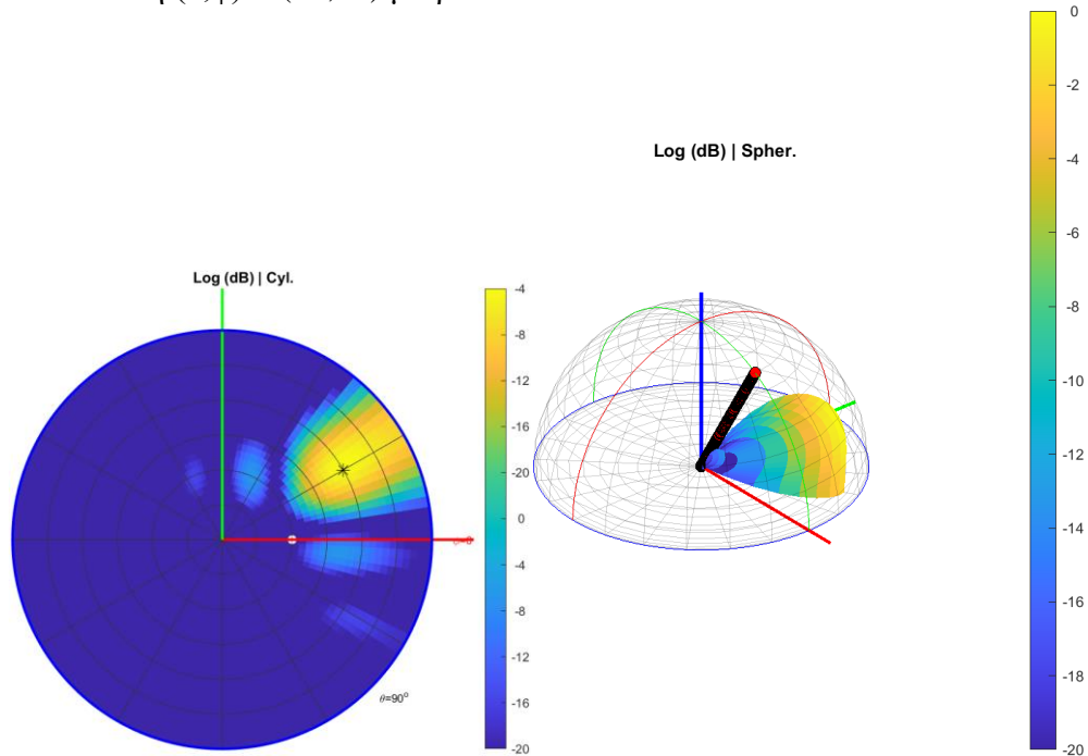
Εικόνα 22 : Πρώτο κομμάτι απόδειξης Beam Splitting FF2FF (Διάγραμμα ακτινοβολίας)
