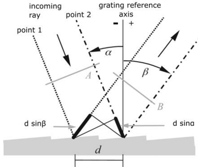
Εικόνα 18: Παράδειγμα Grating
