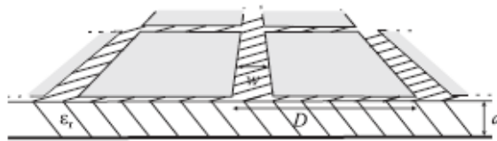
Εικόνα 9: Μια δομή υψηλής αντίστασης που αποτελείται από μια σειρά από patches πάνω από μια διηλεκτρική πλάκα με μεταλλική βάση.
