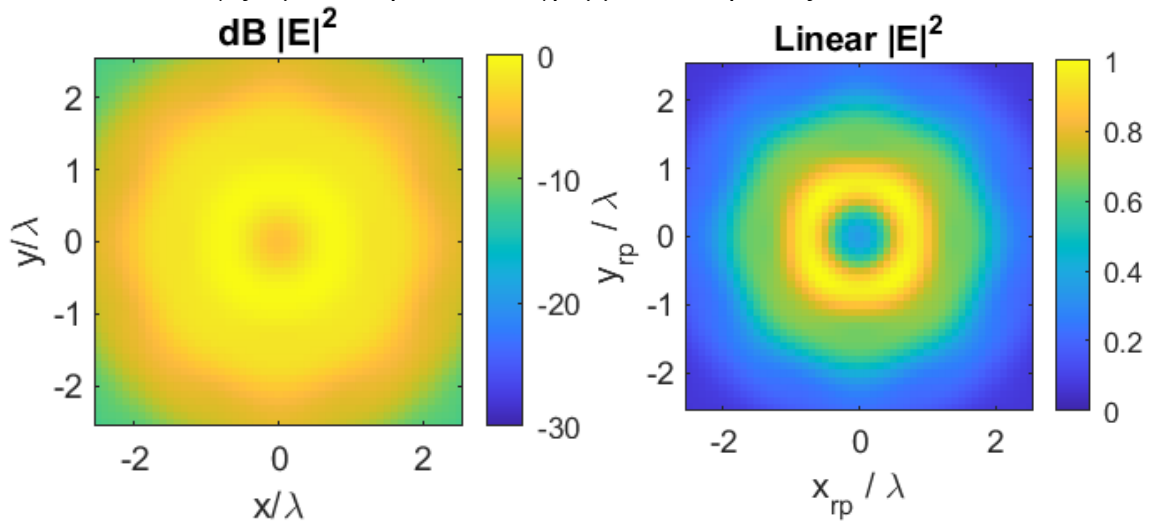
Εικόνα 44: Διάγραμμα ακτινοβολίας για σφαιρικό κύμα στο κοντινό πεδίο
