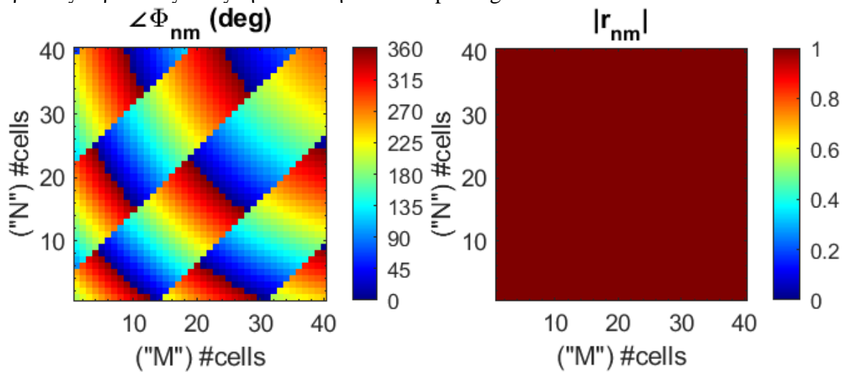
Εικόνα 34: Προφίλ φάσης και πλάτους M/E για σφαιρικό προσπίπτον για Beam Splitting
