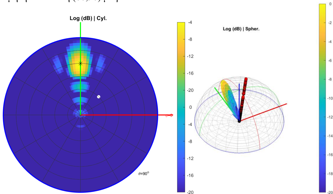
Εικόνα 51 : Διάγραμμα ακτινοβολίας για beam steering επίπεδου κύματος σε (\theta, \varphi)=(60,90)
