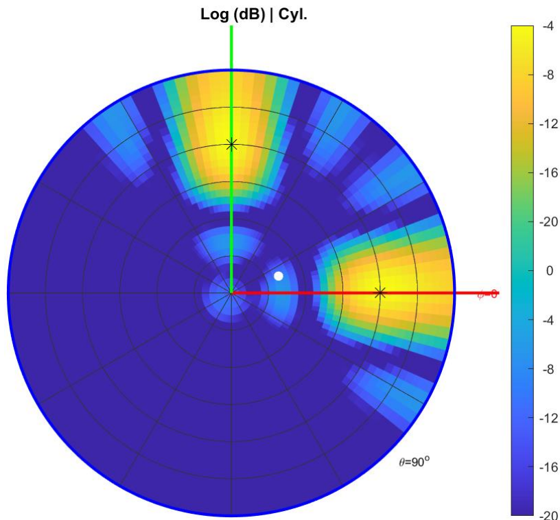
Εικόνα 35: Διάγραμμα ακτινοβολίας σφαιρικού κύματος για Beam Splitting
