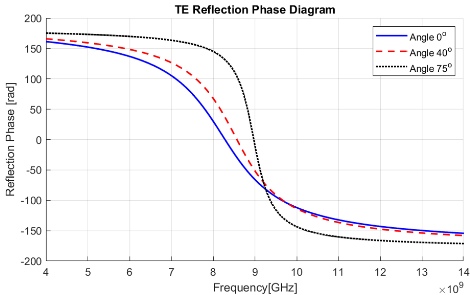
Εικόνα 10: Διάγραμμα φάσης ανάκλασης για TE-πολωμένα προσπίπτοντα πεδία για επιφάνεια υψηλής αντίστασης που αποτελείται από χωρητικές ταινίες για διαφορετικές γωνίες πρόσπτωσης. Οι παράμετροι της επιφάνειας υψηλής σύνθετης αντίστασης είναι οι εξής: D = 3\text{mm} , w = 0,4\text{mm} , d = 15\text{mm} , και \epsilon_r = 10.2
