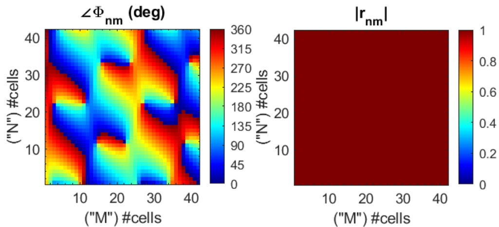
Εικόνα 60: Φάση και πλάτος μεταεπιφάνειας για διάσπαση δέσμης σε 3 λοβούς για επίπεδο προσπίπτον
