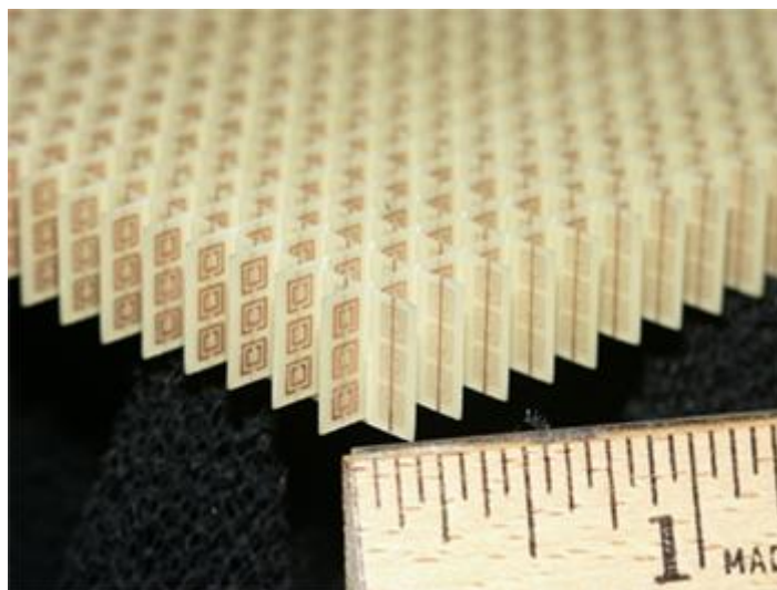
Εικόνα 2: Split-ring resonators του John Pendry
