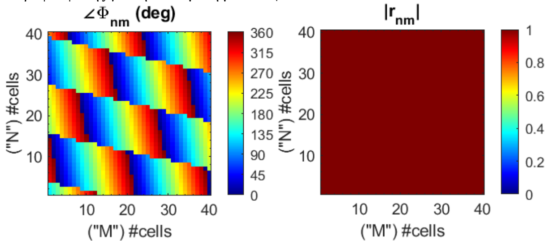
Εικόνα 58: Φάση και Πλάτος μεταεπιφάνειας για beam splitting 2 λοβών επίπεδου κύματος σε (\theta, \varphi)=(45,90) και (\theta, \varphi)=(30,240)
