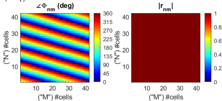
Εικόνα 50: Υπολογισμένο προφίλ φάσης grating και standard πλάτος μεταεπιφάνειας
