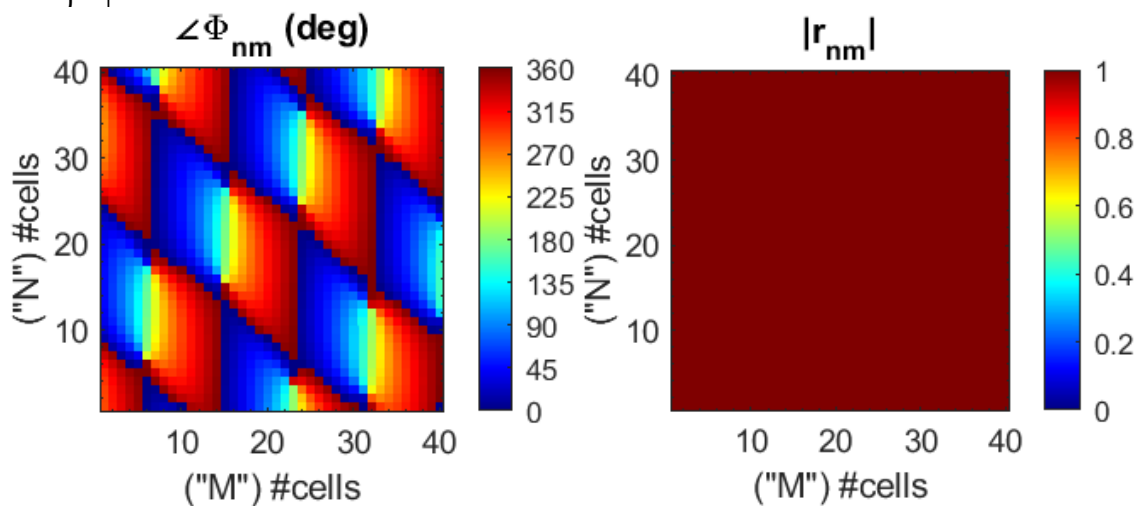
Εικόνα 27: Φάση και Πλάτος Beam Splitting σε 3 λοβούς
