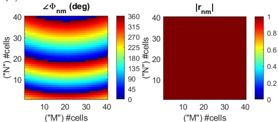
Εικόνα 32: Φάση και πλάτος επιπέδων μονής δέσμης σφαιρικού
