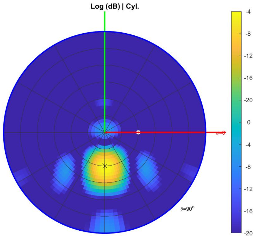
Εικόνα 24: Δεύτερο κομμάτι απόδειξης Beam Splitting FF2FF (Διάγραμμα ακτινοβολίας)
