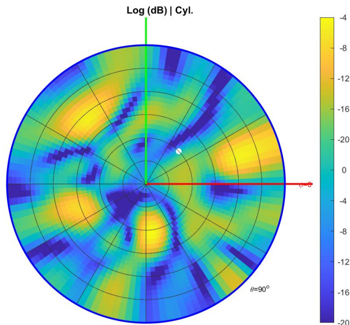
Εικόνα 65: Διάγραμμα ακτινοβολίας για diffused scattering επίπεδου κύματος
