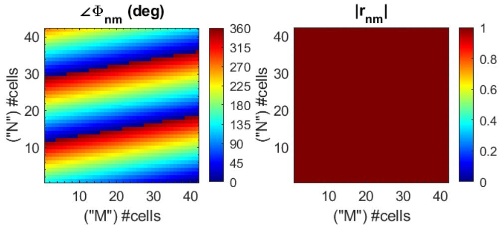
Εικόνα 52: Φάση και πλάτος επίπεδου κύματος ανακατεύθυνσης δέσμης
