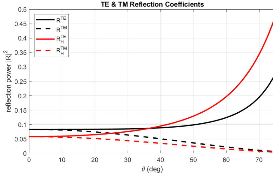
Εικόνα 8: Ο συντελεστής ανάκλασης TE- TM έναντι της γωνίας πρόσπτωσης για μια σειρά από τετράγωνα patches. Οι διαστάσεις του πλέγματος είναι οι εξής: D = /15 και w = D/15 . Η RH αντιστοιχεί στα αποτελέσματα σύμφωνα με το μοντέλο του C. L. Holloway
