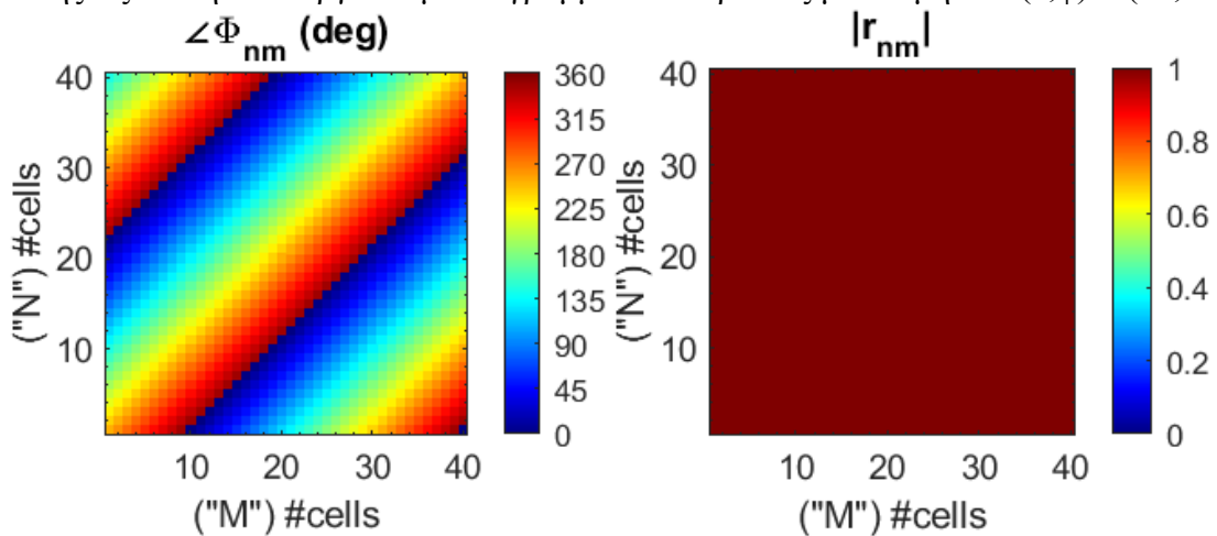
Εικόνα 23: Δεύτερο κομμάτι απόδειξης Beam Splitting FF2FF (Φάση & Πλάτος)
