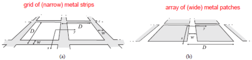
Εικόνα 5: (α) Ένα πλέγμα από ιδανικά αγώγιμες ταινίες σε ομοιογενές μέσο. (β) Συστοιχία patches σε ομοιογενές μέσο. Τα μεταλλικά μέρη έχουν γκρι χρώμα.
