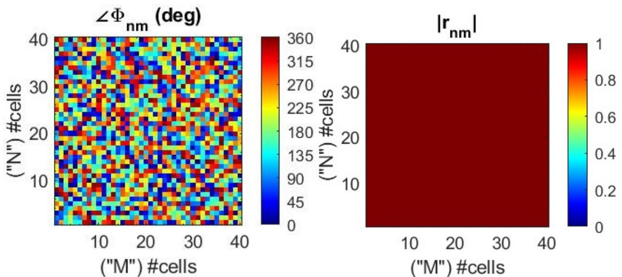
Εικόνα 19: Φάση και πλάτος για Diffused Scattering FF2FF
