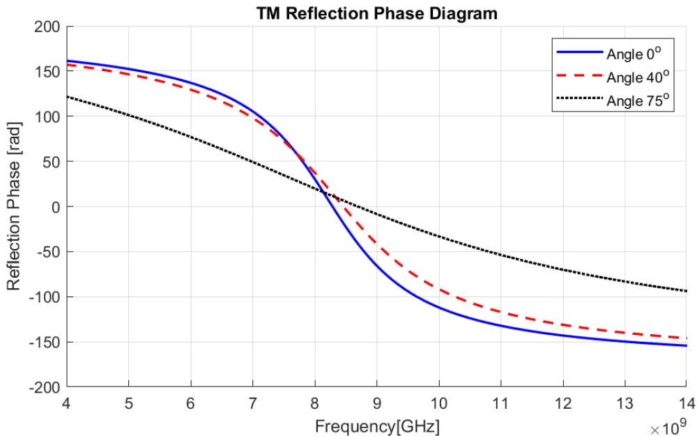
Εικόνα 13: Φάση ανάκλασης για πολωμένο προσπίπτον πεδίο TM για επιφάνεια υψηλής σύνθετης αντίστασης που αποτελείται από τετράγωνα patches για διαφορετικές γωνίες πρόσπτωσης. D=3\text{mm} w=0.4\text{mm} d=0.15\text{mm} \epsilon_r=10.2
