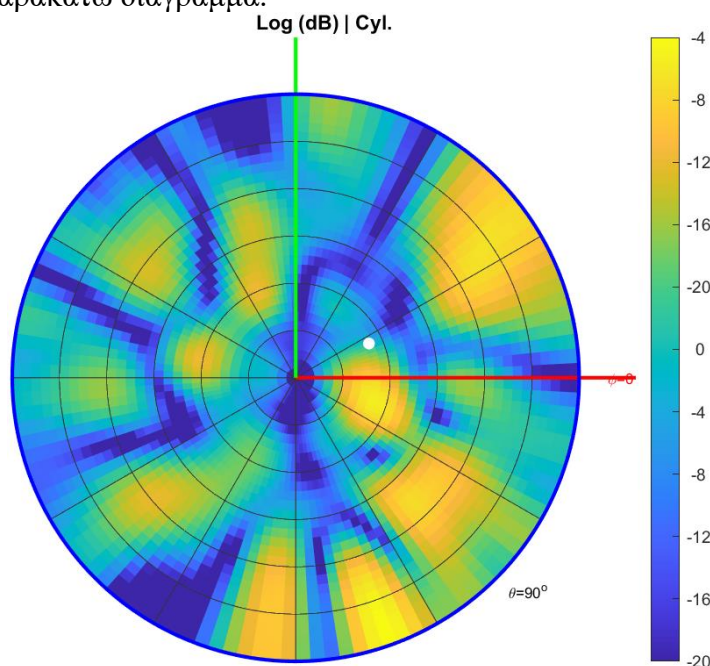
Εικόνα 67: Διάγραμμα ακτινοβολίας για diffused scattering σφαιρικού κύματος
