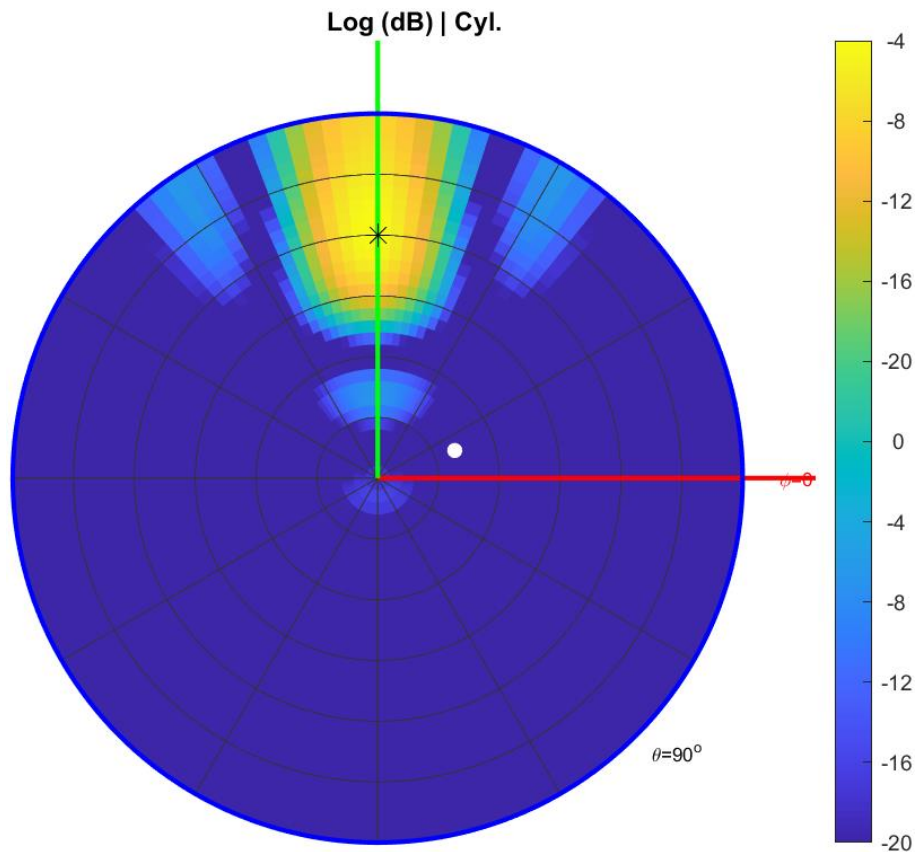
Εικόνα 33: Διάγραμμα ακτινοβολίας επιπλέον μονής δέσμης σφαιρικού
