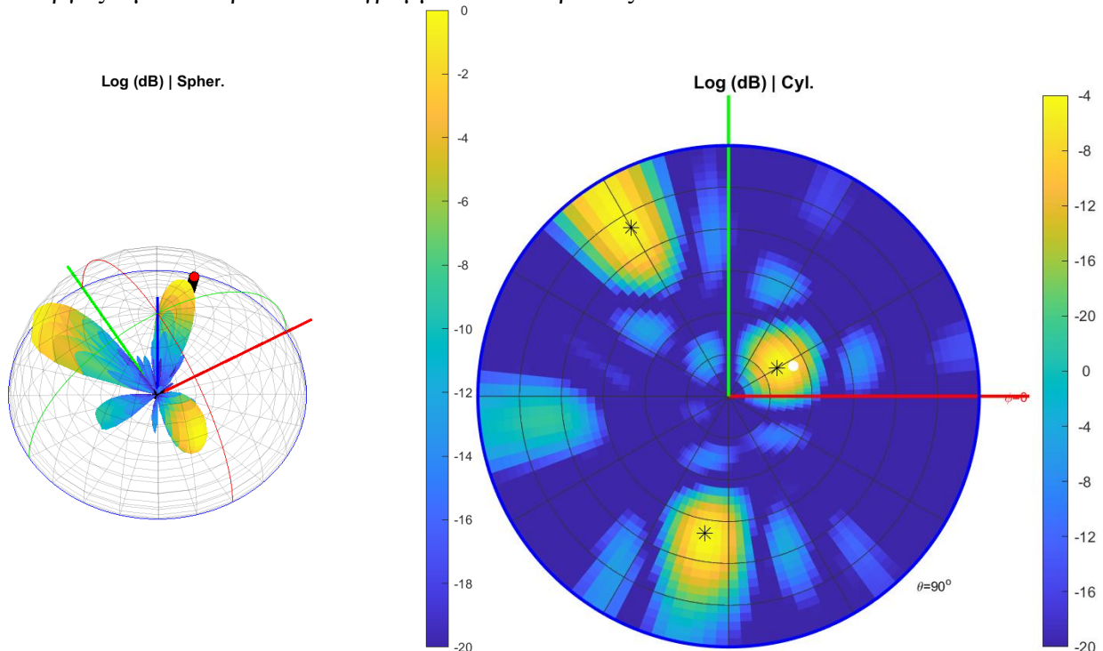
Εικόνα 63: Διάγραμμα ακτινοβολίας για beam splitting 3 λοβών από σφαιρικό κύμα
