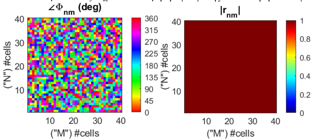
Εικόνα 36: Φάση και πλάτος μεταεπιφάνειας για diffused scattering σφαιρικού προσπίπτοντος
