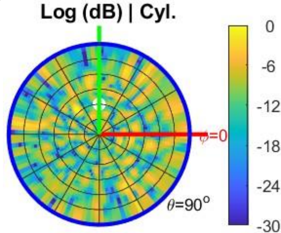
Εικόνα 29: Διάγραμμα ακτινοβολίας για diffused scattering
