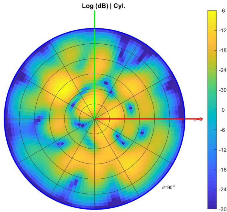
Εικόνα 37: Διάγραμμα ακτινοβολίας για diffused scattering σφαιρικού κύματος
