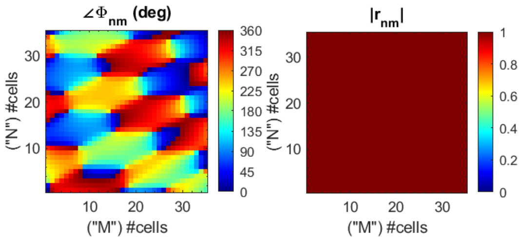
Εικόνα 62: Φάση και πλάτος μεταεπιφάνειας για beam splitting 3 λοβών σφαιρικού κύματος
