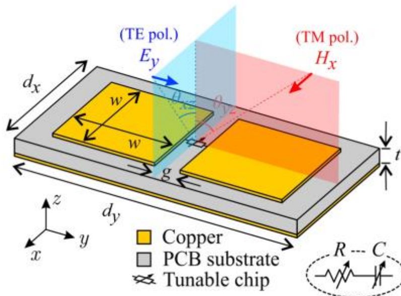
Εικόνα 17: Δομή RIS
