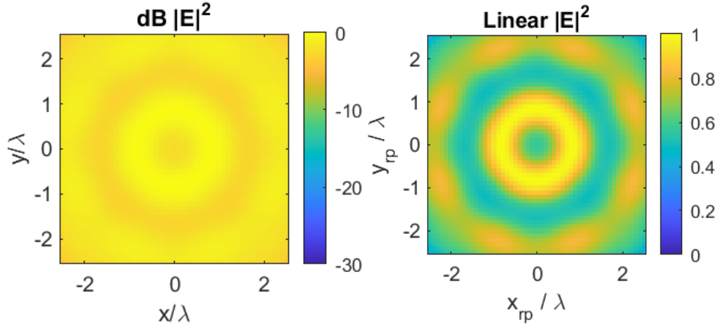
Εικόνα 46: Διάγραμμα ακτινοβολίας spot-diagram για σφαιρικό κύμα
