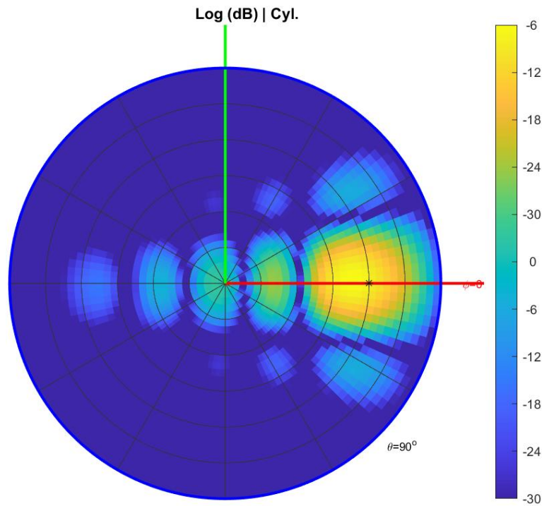
Εικόνα 31: Διάγραμμα ακτινοβολίας σφαιρικού κύματος για Beam Steering
