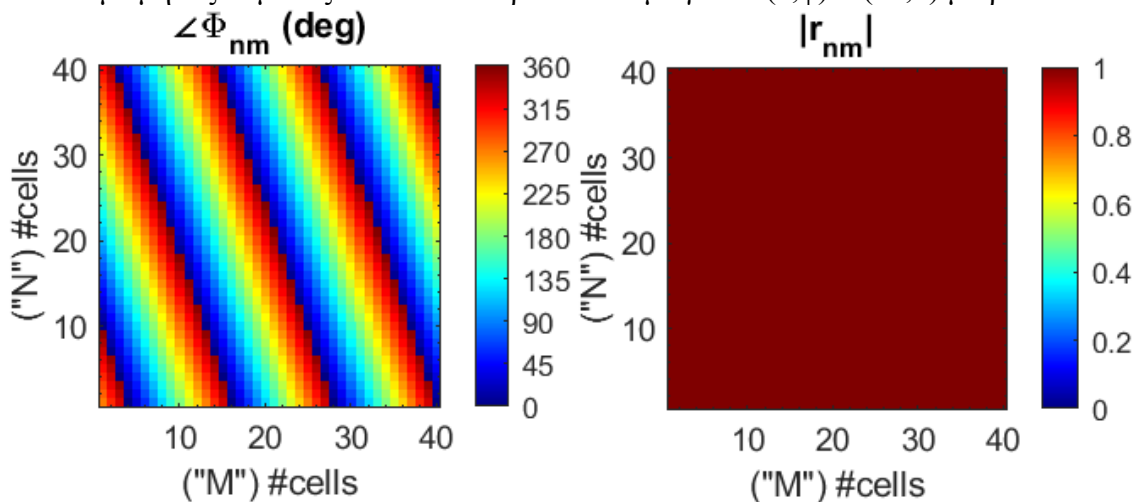
Εικόνα 21: Πρώτο κομμάτι απόδειξης Beam Splitting FF2FF (Φάση & Πλάτος)
